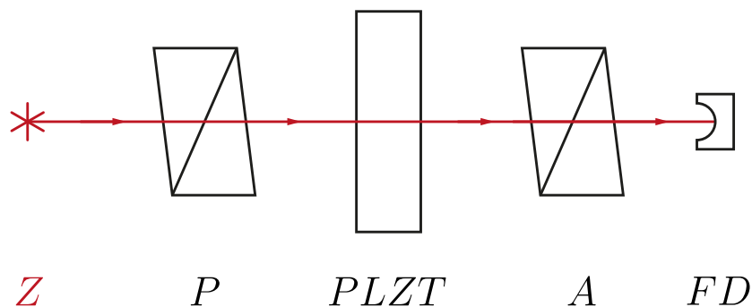
Obrázek 1: Schéma měřicí aparatury
